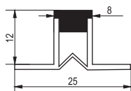
■ PVC dilatacioni profil za fugne.
