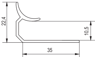
■ Aluminijumski profil za unutrašnji ugao.
