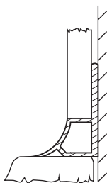
■ Završni PVC profil za spojeve kada i keramičkih pločica
