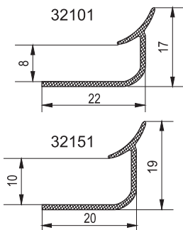
■ PVC profil sa elastičnim završetkom - unutrašnji ugao.
