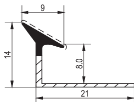
■ PVC profil sa elastičnim završetkom - unutrašnji ugao.
